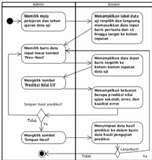
Gambar 8. Rancangan Activity Diagram Uji JST
